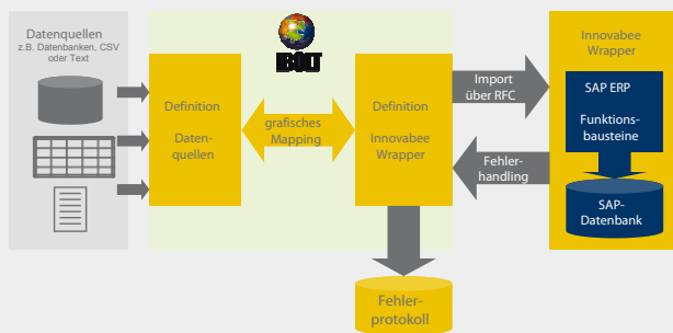
Standard-Migrationstool von Innovabee
