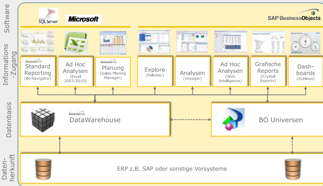
Überblick BI-Lösungen von Innovabee
