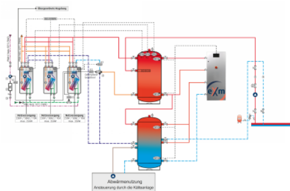
Das Anschlussschema zeigt die beiden Speicher, die sich zu einem großen Schichtspeicher-System ergänzen, die eXergiemaschine (rechts) zum Optimieren der Temperaturschichtung sowie die Dreier-Kaskade an Frischwasserstationen (links), die Warmwasser im hygienischen Durchlaufprinzip bereitstellen. (Bild: BMS)
